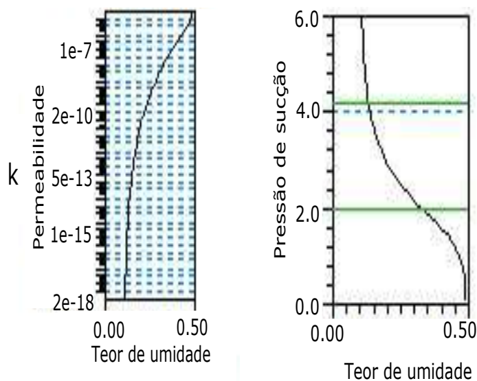
Figura 7.2: Curvas de condutividade hidráulica e de retenção da areia fina
