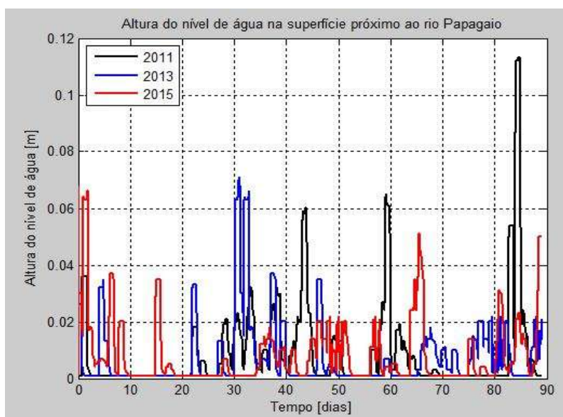
Figura 9.11: Lâmina de água na superfície próximo ao rio Papagaio
