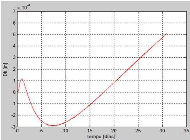
Figura 6.5: Cálculo do erro entre as duas soluções
