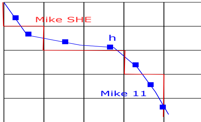
Figura 5.2: Representação do mapeamento da rede hidrográfica feito pelo MIKE SHE
