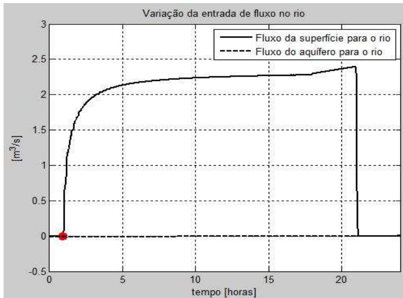
Figura 7.8: Acoplamento do Mike 11 com a zona saturada e a superfície
