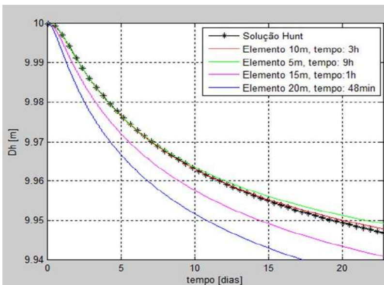
Figura 6.6: Convergência de malhas
