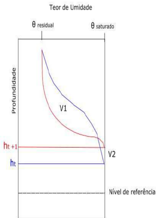
Figura 7.7: Esquema do balanço iterativo entre a zona não saturada e saturada
