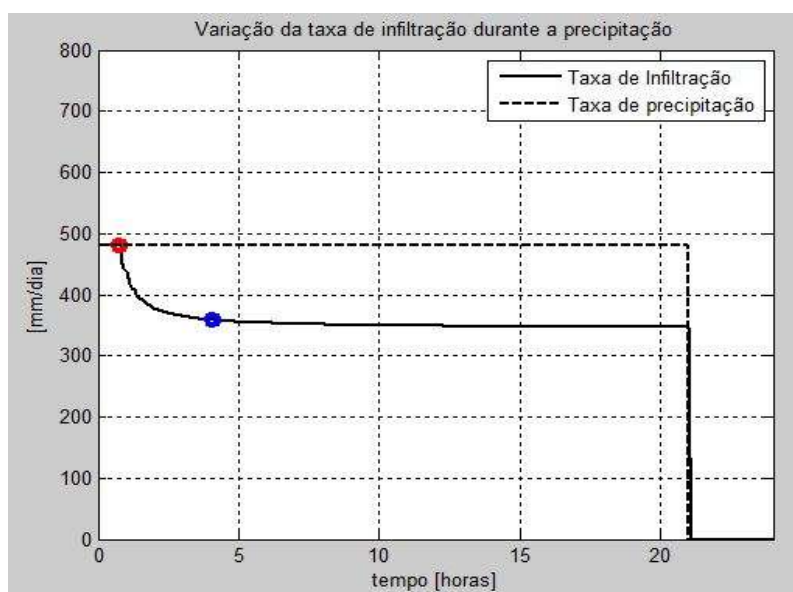
Figura 7.3: Variação da taxa de infiltração
