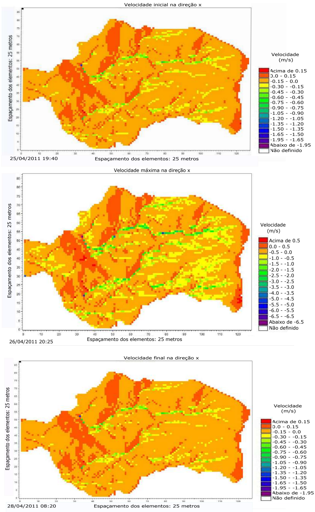
Figura 9.7: Mapa de velocidades em evento de precipitação em 2011
