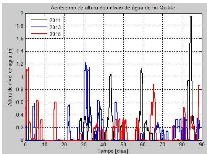
Figura 9.16: Nível de água do rio Quitite
