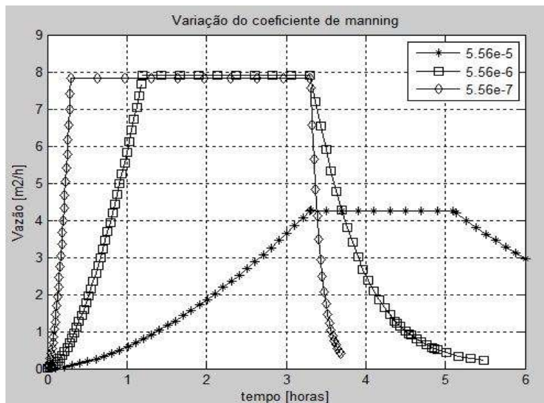
Figura 6.11: Hidrograma para diferentes coeficientes de Manning
