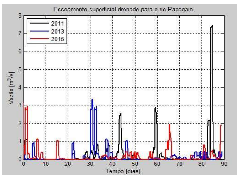
Figura 9.13: Vazão da superfície para o rio Papagaio
