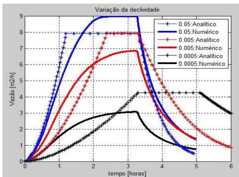
Figura 6.10: Comparação entre a solução analítica e numérica variando a declividade
