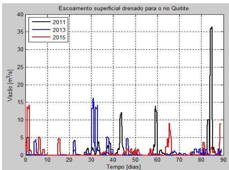
Figura 9.14: Vazão da superfície para o rio Quitite
