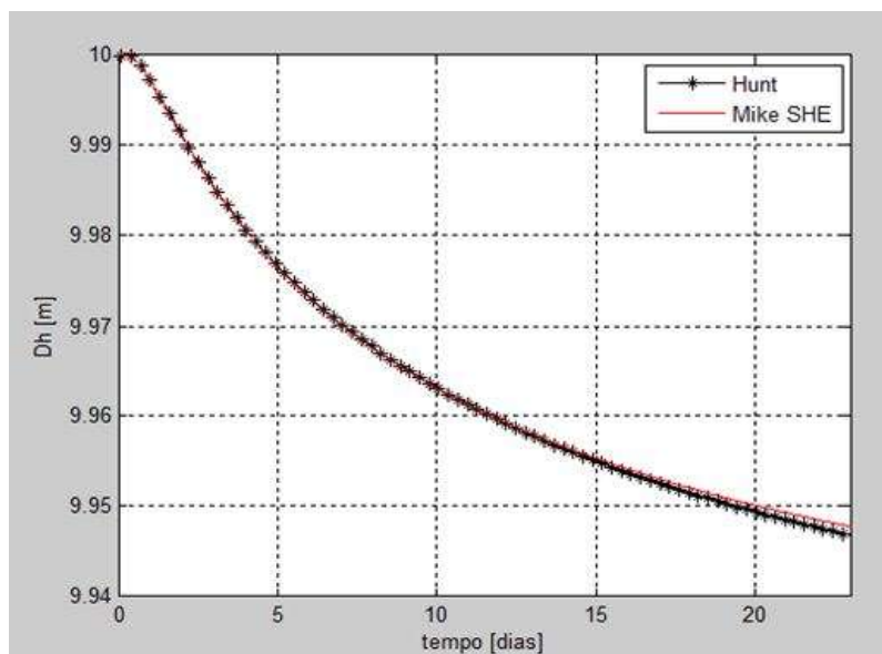
Figura 6.3: Comparação entre a solução analítica proposta por Hunt(1999) e pelo programa Mike SHE
