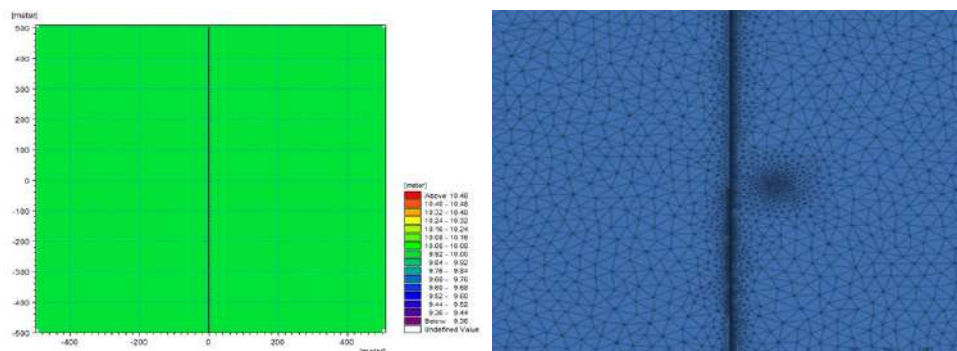
Figura 6.7: Malha de elementos finitos gerada pelo Mike SHE e Feflow
