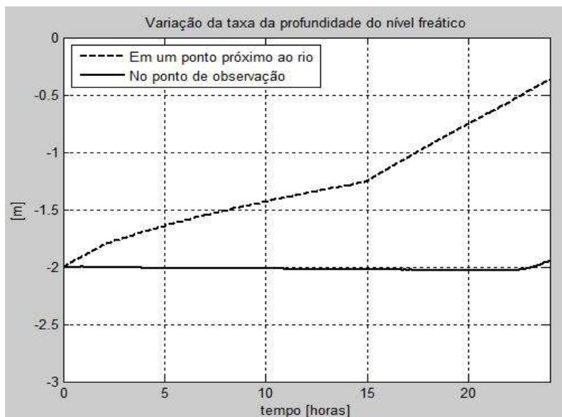
Figura 7.6: Profundidade do nível freático
