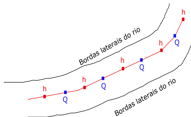
Figura 5.4: Malha Computacional definida no MIKE 11
