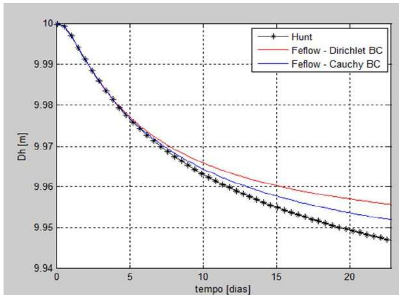
Figura 6.4: Comparação entre a solução analítica proposta por Hunt(1999) e os resultados obtidos pelo programa Feflow com suas respectivas condições de contorno
