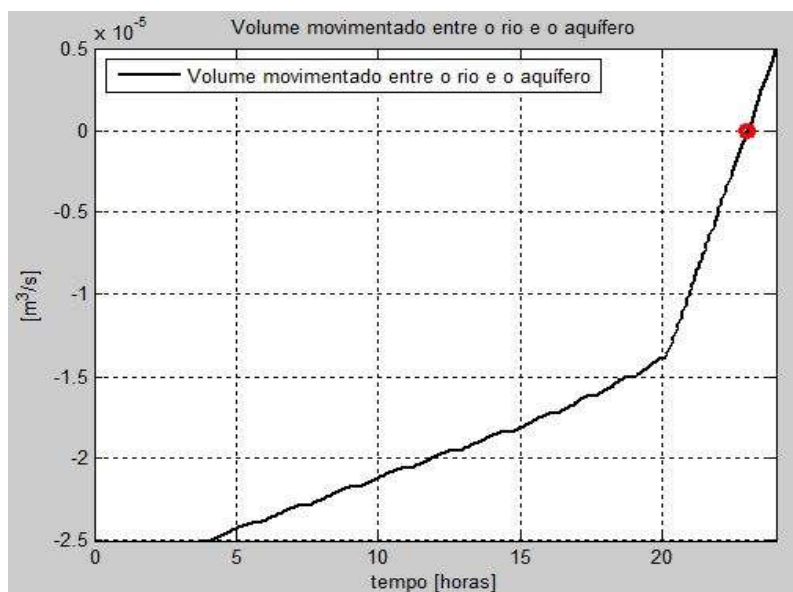
Figura 7.9: Volume movimentado entre a zona saturada e o rio
