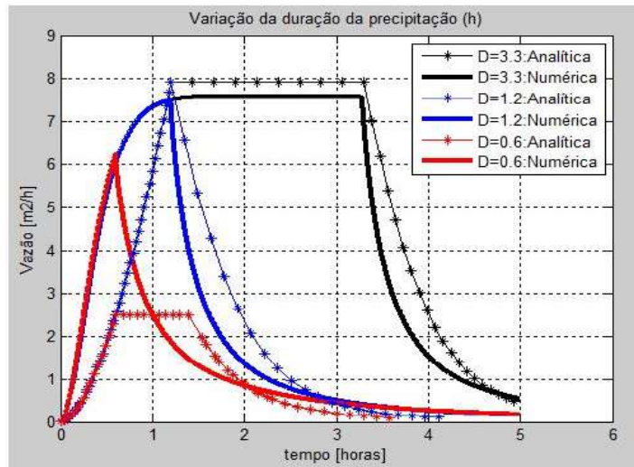
Figura 6.16: Comparação entre a solução analítica e numérica variando o tempo de precipitação
