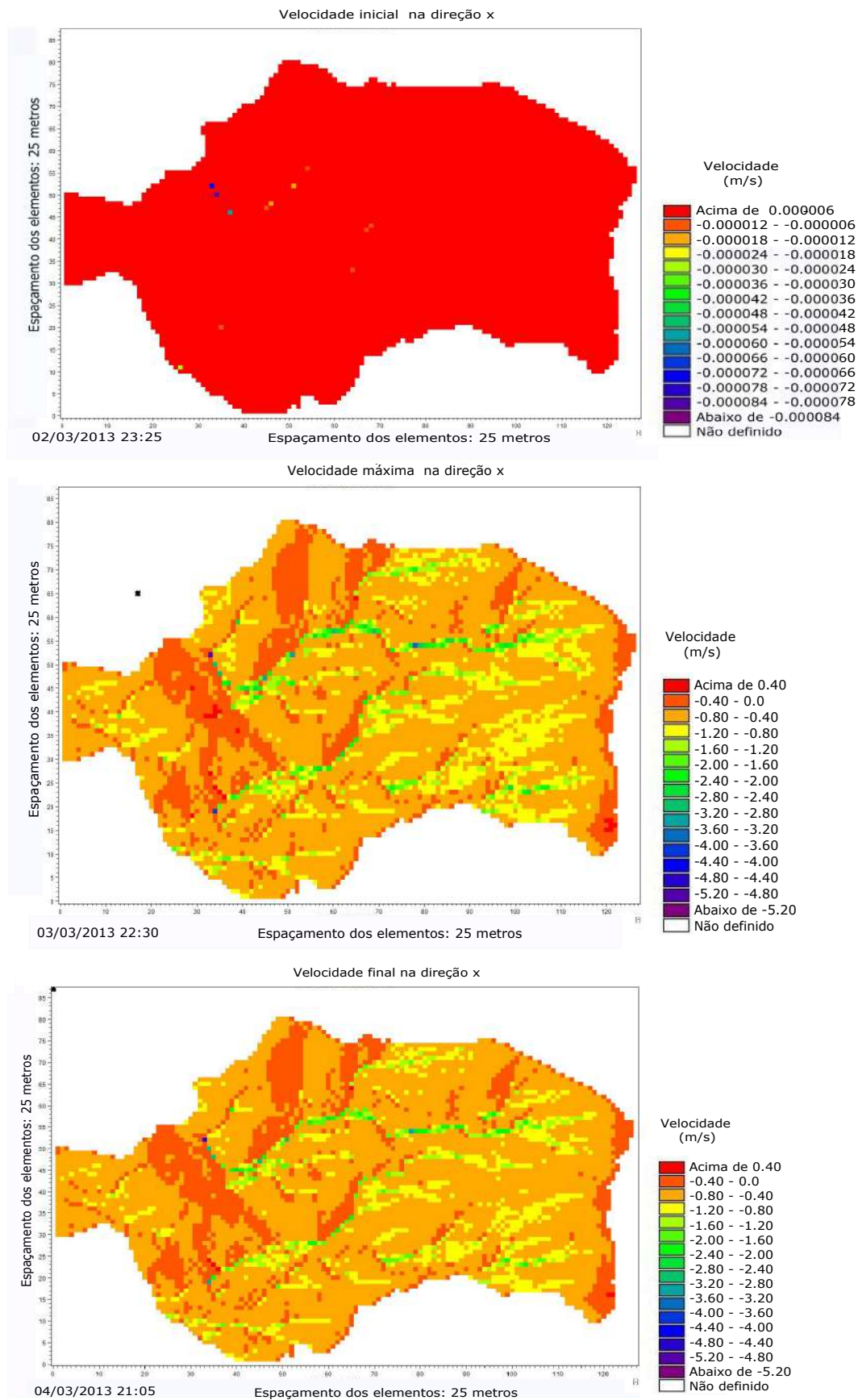
Figura 9.8: Mapa de velocidades em evento de precipitação em 2013
