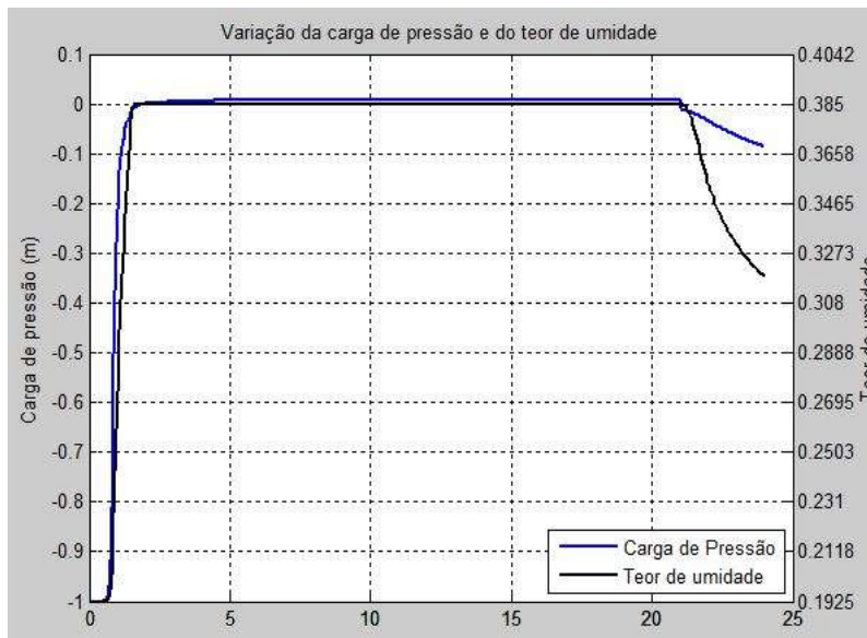
Figura 7.5: Zona não saturada
