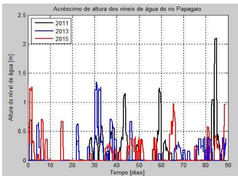
Figura 9.15: Nível de água do rio Papagaio
