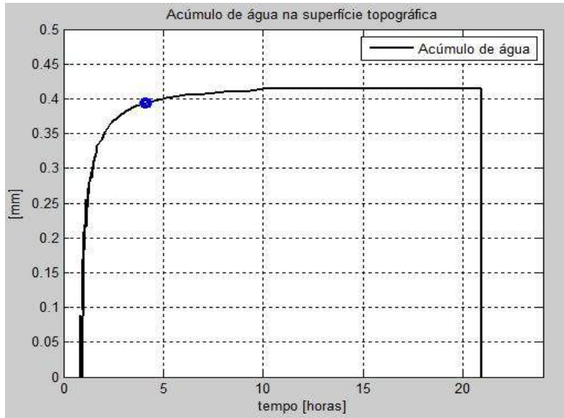
Figura 7.4: Acúmulo de água na superfície
