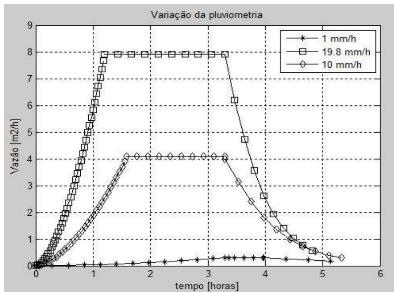
Figura 6.13: Hidrograma para diferentes intensidades de precipitação
