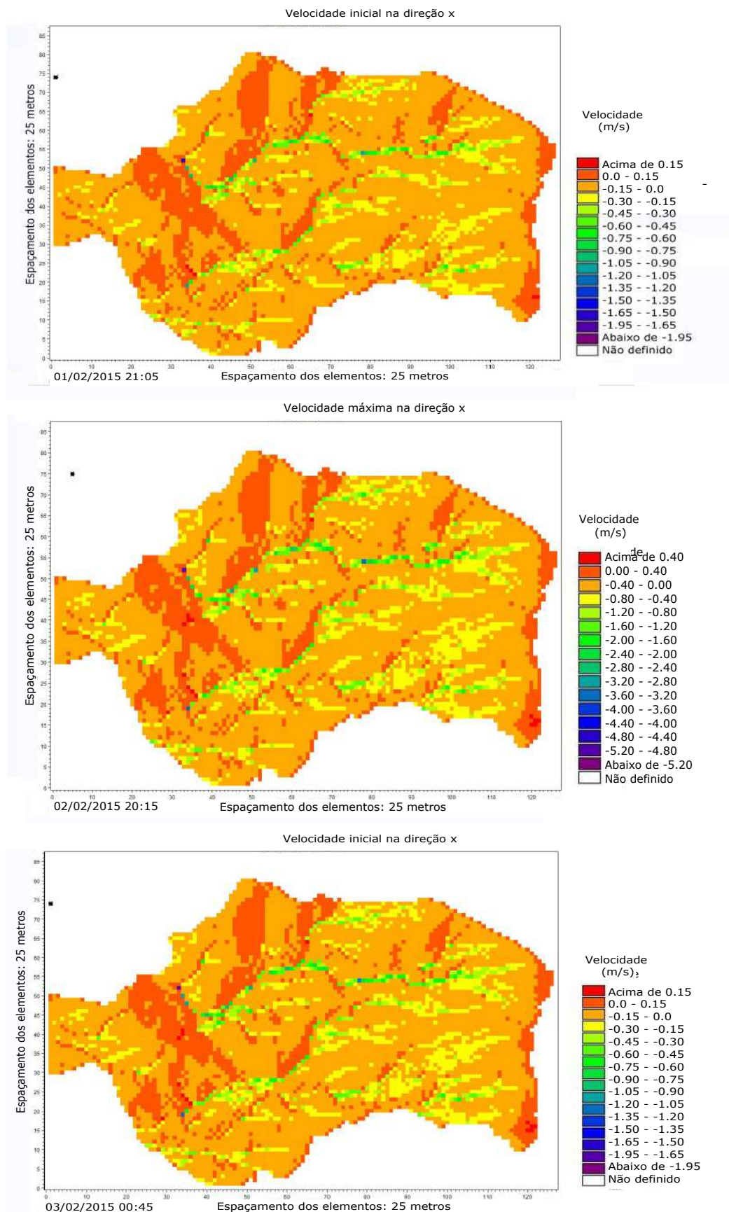
Figura 9.9: Mapa de velocidades em evento de precipitação em 2015
