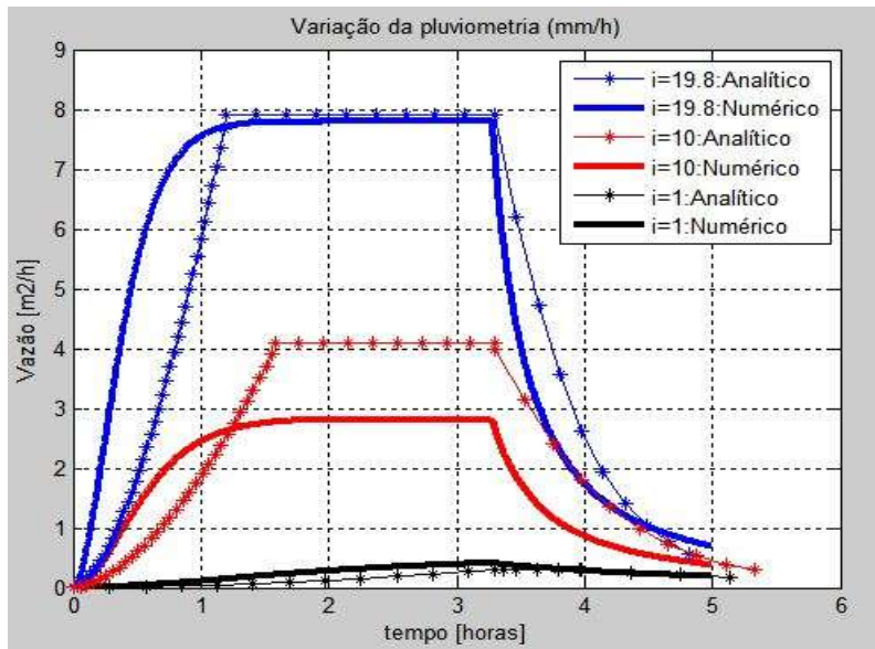
Figura 6.14: Comparação entre a solução analítica e numérica variando a intensidade de precipitação
