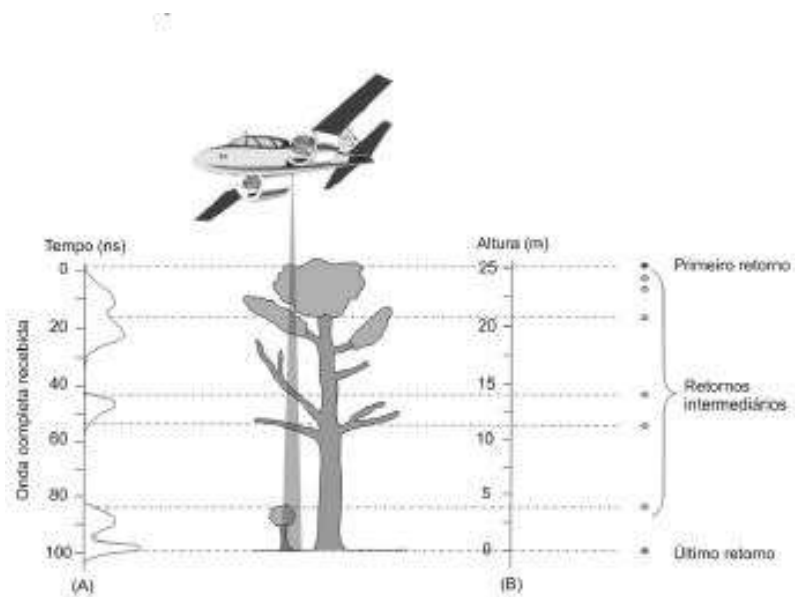
Figura 8.5: Desenho esquemático do levantamento aéreo LIDAR [52]
