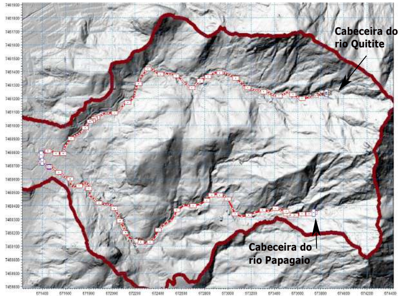
Figura 8.6: Acoplamento da superfície topográfica com os rios
