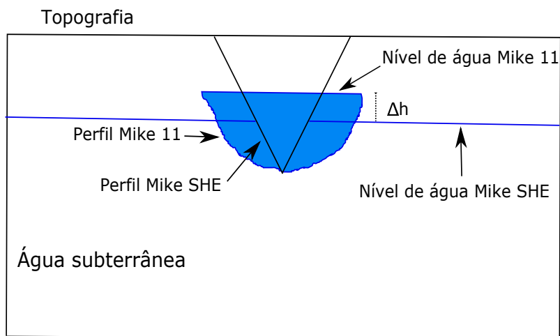
Figura 5.3: Leitura da seção do rio pelo Mike SHE
