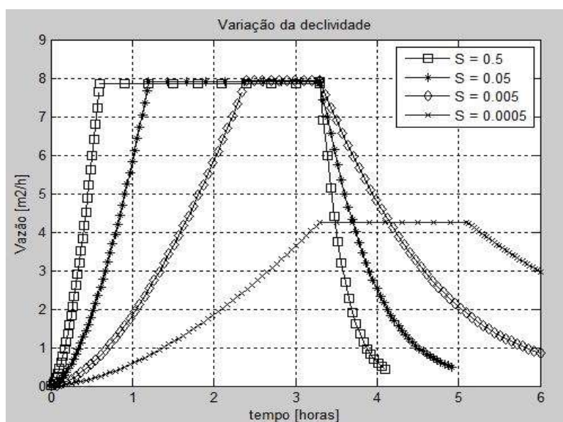
Figura 6.9: Hidrogramas para declividades diferentes
