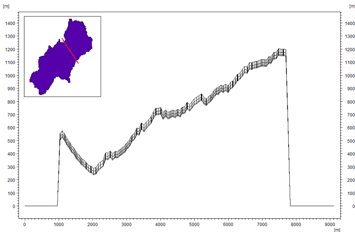
Figura 31 - Corte longitudinal da zona saturada do modelo
