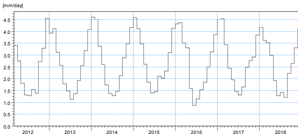
Figura 18 - Valores diários de evapotranspiração de referência no C0 (cenário com as unidades de conservação).
