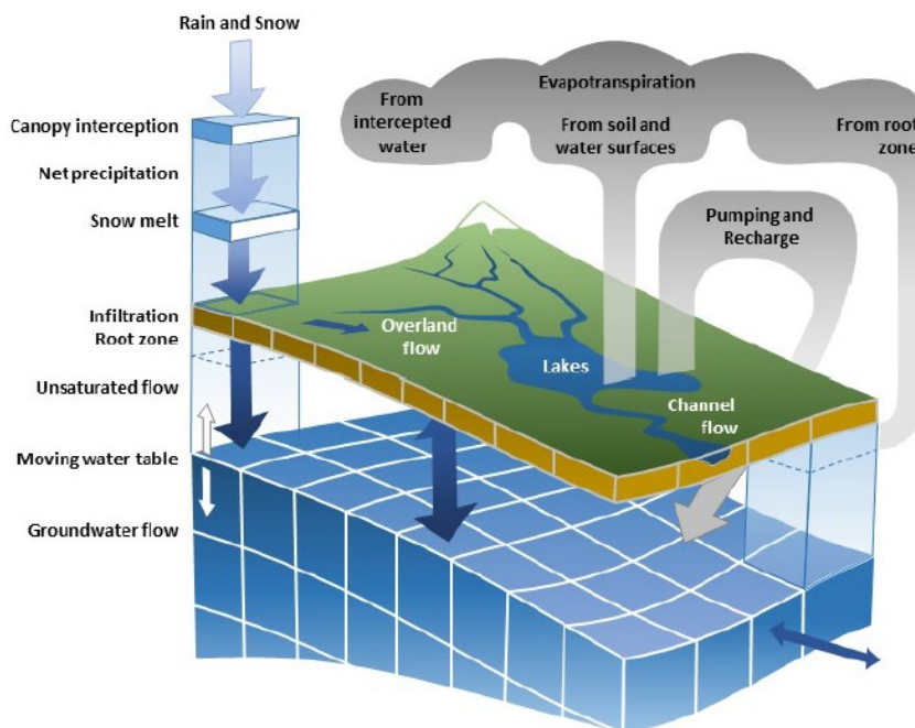
Figura 9 - Processos hidrológicos do módulo de movimento de água do MIKE SHE.
