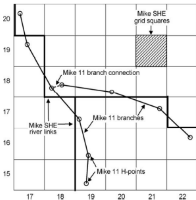
Figura 10 - Esquema de acoplamento entre MIKE SHE e MIKE 11.
