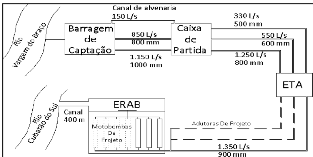
Figura 3 - Esquema de captação e adução de água bruta dos rios Vargem do Braço e Cubatão do Sul.
